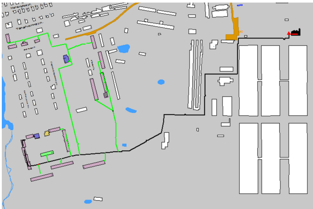
Рисунок Ошибка! Текст указанного стиля в документе отсутствует..231 Результат гидравлического расчета - расчетный путь теплоносителя от котельной Заслонова, 20 до ПТ-Береговая,16
