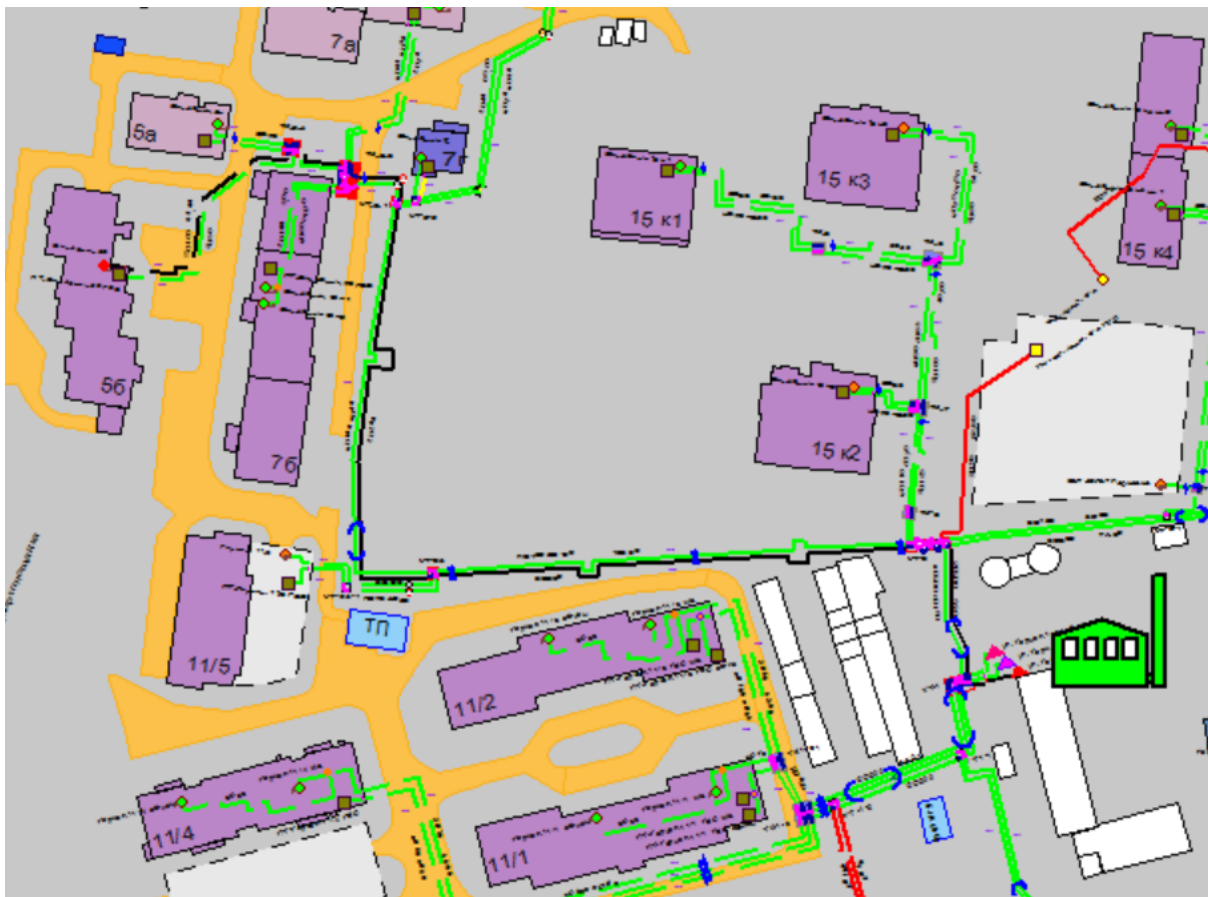
Рисунок Ошибка! Текст указанного стиля в документе отсутствует..41 Результат гидравлического расчета - расчетный путь теплоносителя от котельной Горная, 13 до ПТ-Окт.40лет,56
