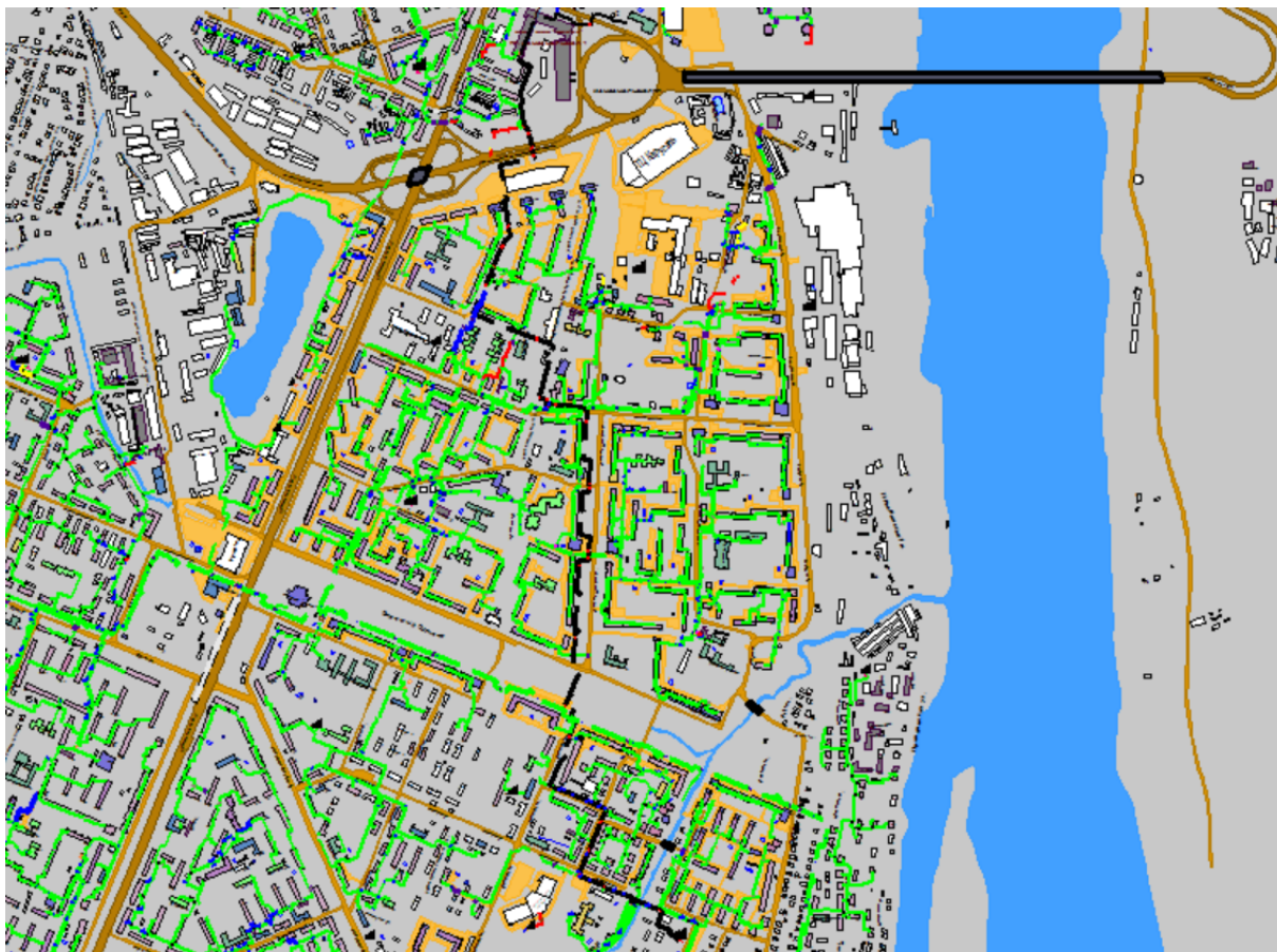
Рисунок Ошибка! Текст указанного стиля в документе отсутствует. 65 Результат гидравлического расчета - расчетный путь теплоносителя от котельной Заводская, 19 до ПТ-Комсом.пл,3
