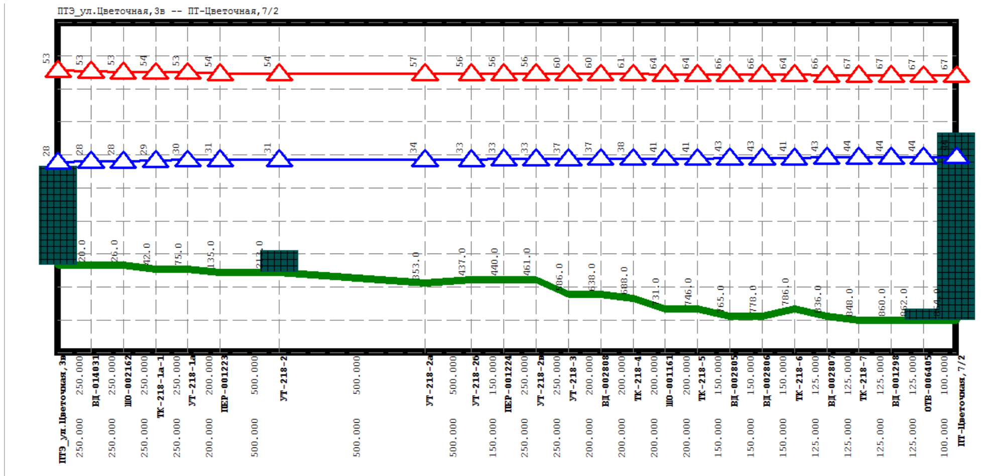
Рисунок Ошибка! Текст указанного стиля в документе отсутствует..48 Результат гидравлического расчета - график гидравлических режимов по пути теплоносителя от котельной Цветочная, 3-а до ПТ-Цветочная,7/2
