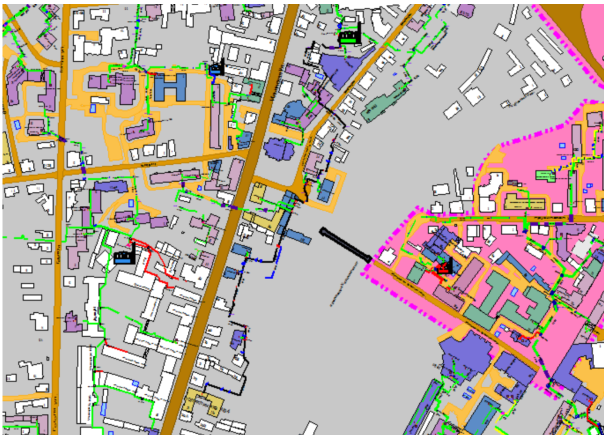
Рисунок Ошибка! Текст указанного стиля в документе отсутствует..23 Результат гидравлического расчета - расчетный путь теплоносителя от котельной Плотничный, 11 до ПТ-Ильин,78,78а
