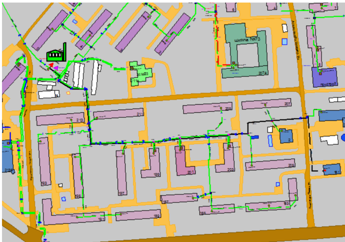
Рисунок Ошибка! Текст указанного стиля в документе отсутствует..79 Результат гидравлического расчета - расчетный путь теплоносителя от котельной Красных Зорь, 4а до ПТ-Моск.ш,181
