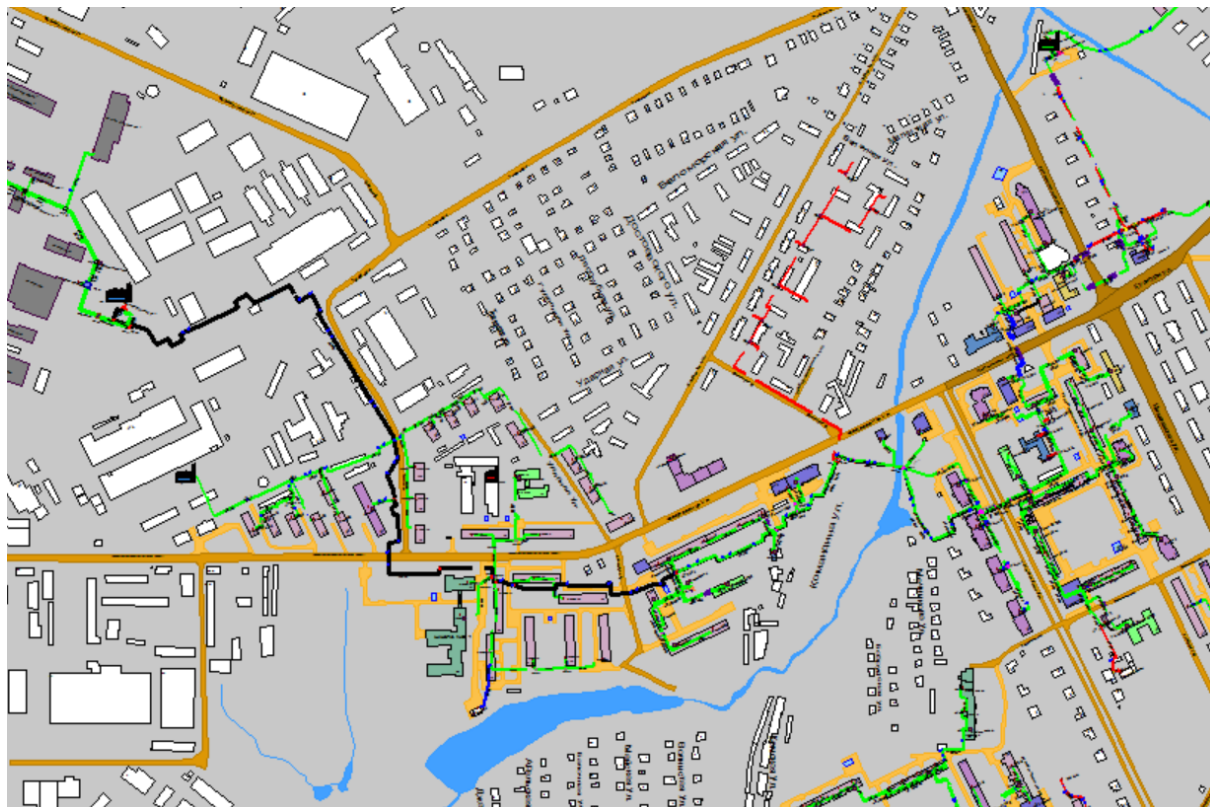
Рисунок Ошибка! Текст указанного стиля в документе отсутствует..213 Результат гидравлического расчета - расчетный путь теплоносителя от котельной Федосеенко, 64 до ПТ-Остров,9
