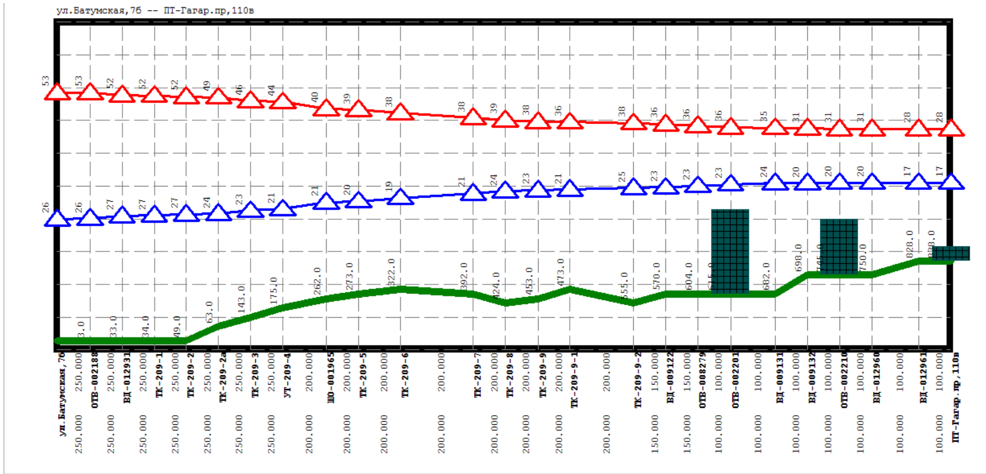
Рисунок Ошибка! Текст указанного стиля в документе отсутствует..28 Результат гидравлического расчета - график гидравлических режимов по пути теплоносителя от котельной Углова, 7 до ПТ-Гагар. пр, 110в
