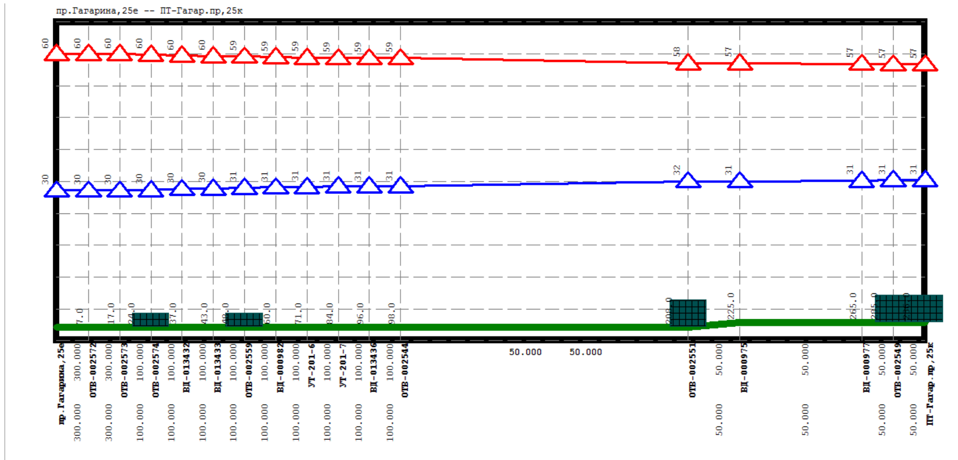
Рисунок Ошибка! Текст указанного стиля в документе отсутствует..56 Результат гидравлического расчета - график гидравлических режимов по пути теплоносителя от котельной Гагарина, 25-е до ПТ-Гагар.пр,25к
