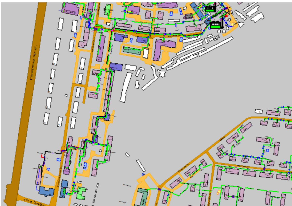
Рисунок Ошибка! Текст указанного стиля в документе отсутствует..223 Результат гидравлического расчета - расчетный путь теплоносителя от котельной Батумская, 7-6 до ПТ-Гагар.пр,146
