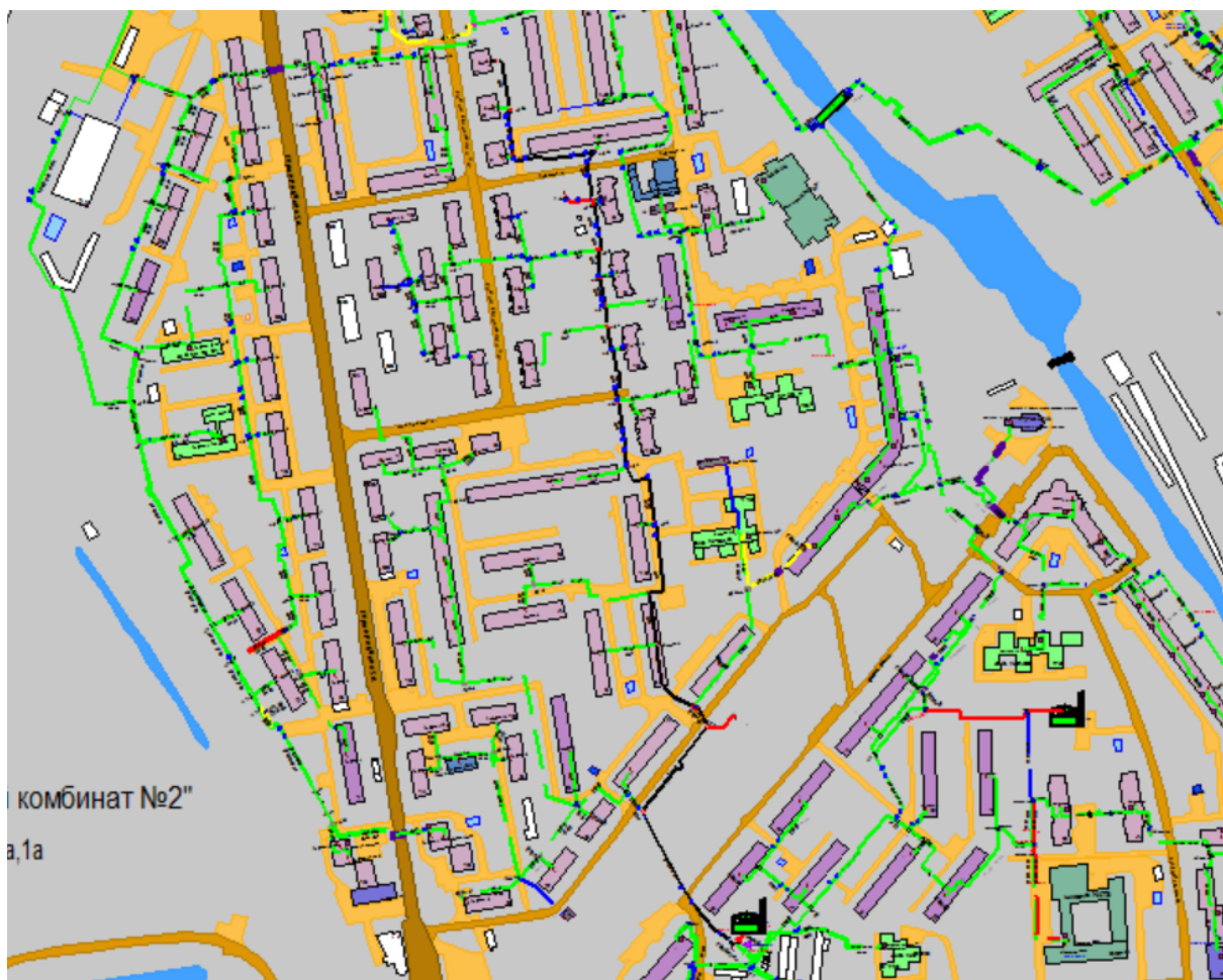
Рисунок Ошибка! Текст указанного стиля в документе отсутствует..77 Результат гидравлического расчета - расчетный путь теплоносителя от котельной Красных Зорь, 4а до ПТ-Давыд,11
