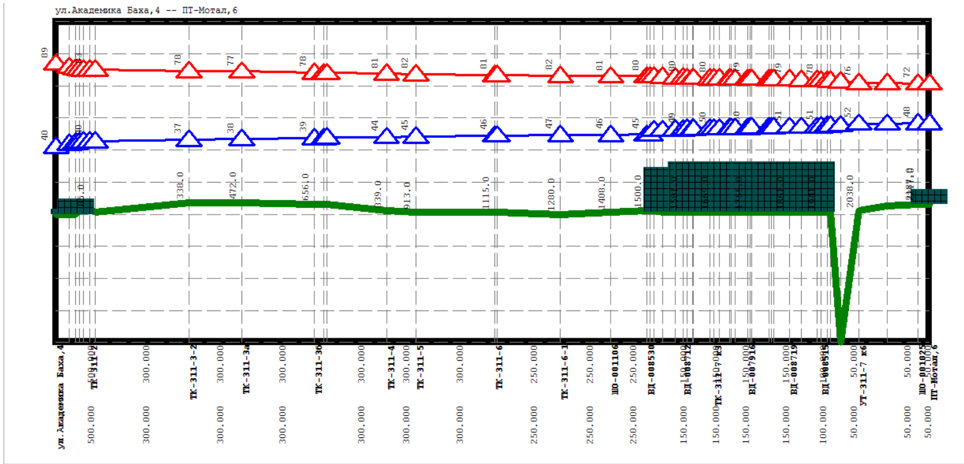
Рисунок Ошибка! Текст указанного стиля в документе отсутствует..8 Результат гидравлического расчета - график гидравлических режимов по пути теплоносителя от котельной Академика Баха, 4-а до ПТ-Мотал,6
