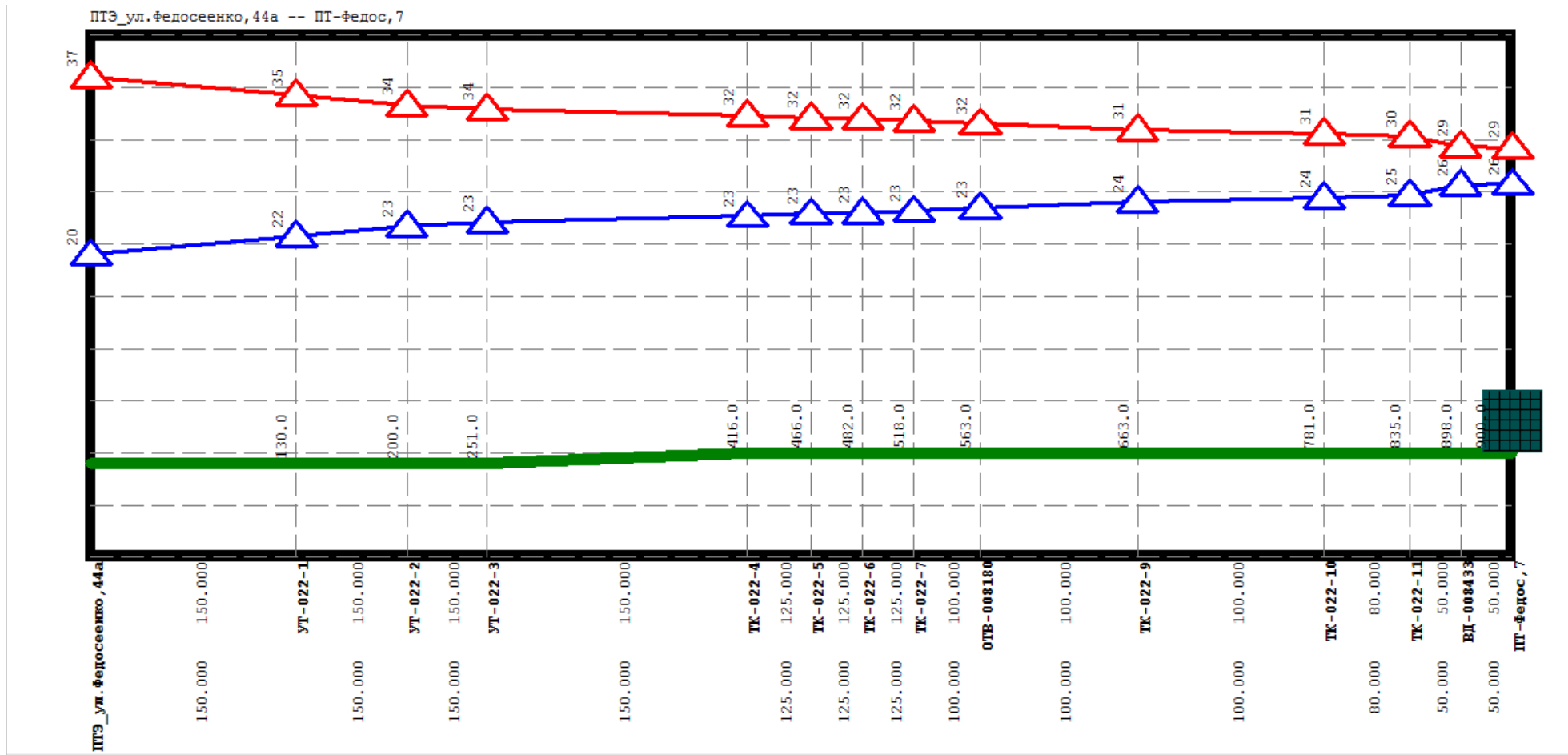
Рисунок Ошибка! Текст указанного стиля в документе отсутствует..210 Результат гидравлического расчета - график гидравлических режимов по пути теплоносителя от котельной Федосеенко, 44а до ПТ-Федос,7
