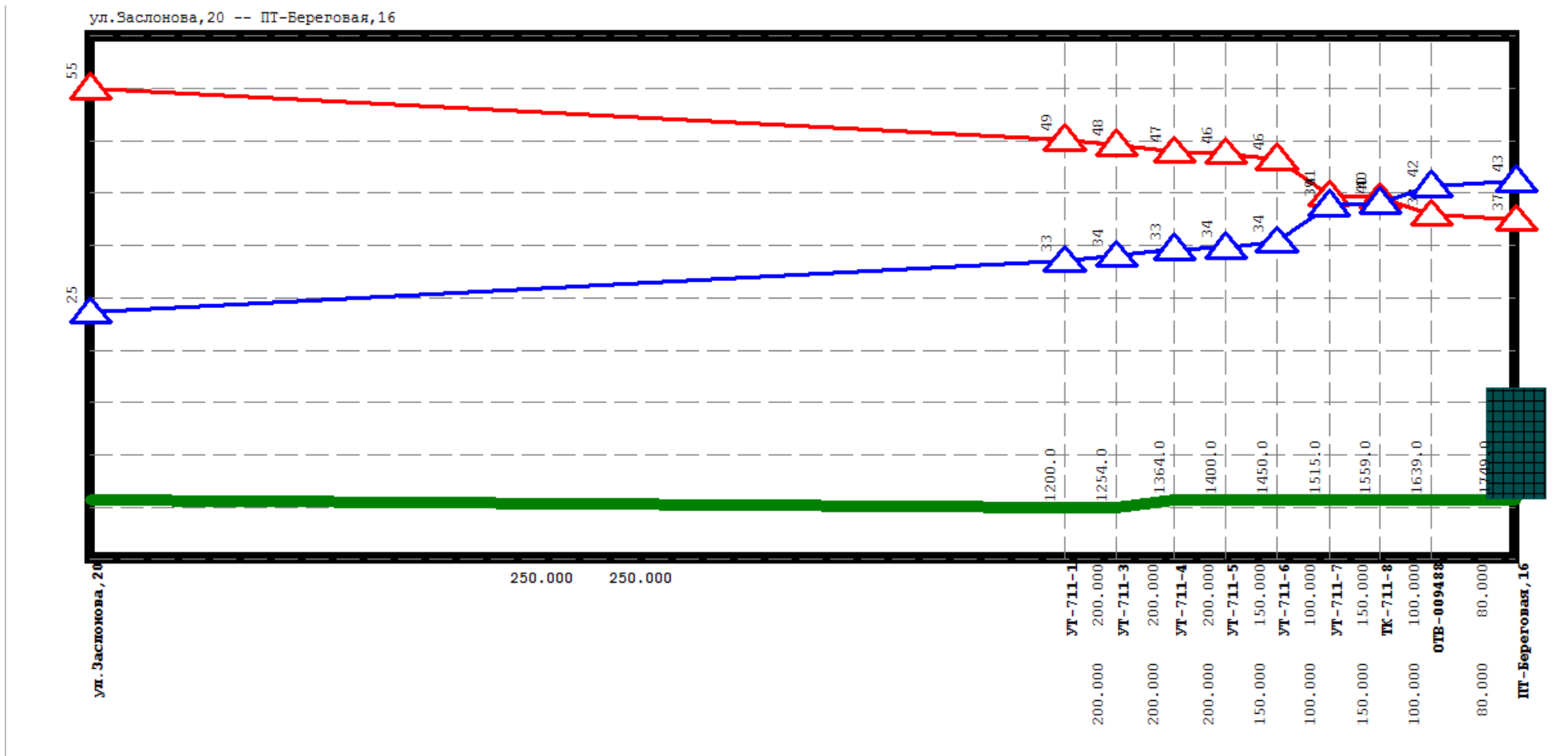
Рисунок 232 Результат гидравлического расчета - график гидравлических режимов по пути теплоносителя от котельной Заслонова, 20 до ПТ-Береговая,16
