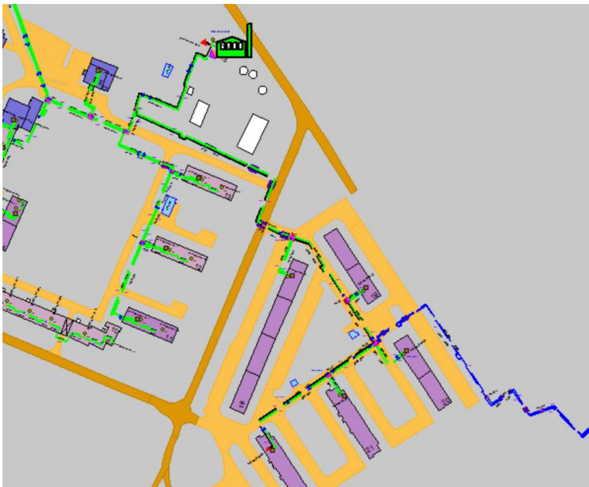
Рисунок Ошибка! Текст указанного стиля в документе отсутствует..45 Результат гидравлического расчета - расчетный путь теплоносителя от котельной 40 лет Победы, 15 до ПТ-Победы 40лет,22
