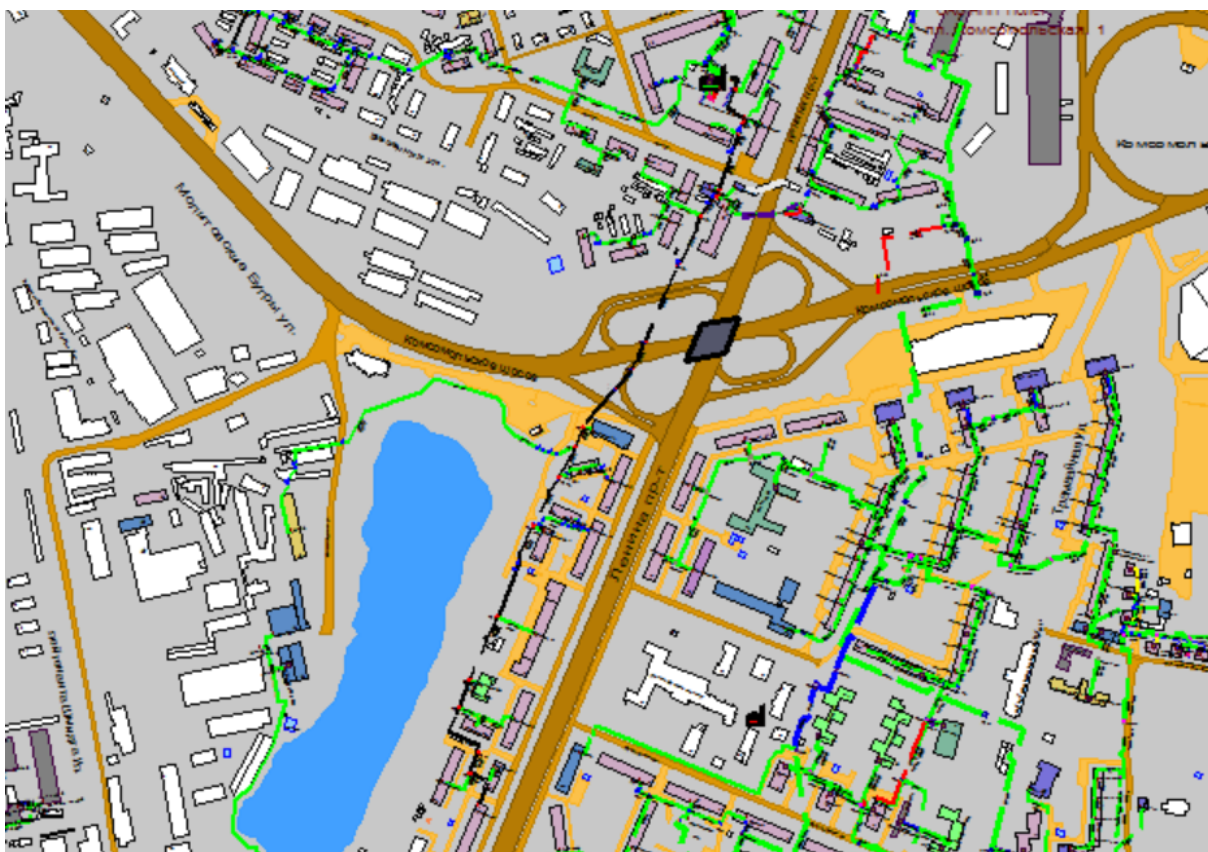
Рисунок Ошибка! Текст указанного стиля в документе отсутствует..15 Результат гидравлического расчета - расчетный путь теплоносителя от котельной пр. Ленина, 5-а до ПТ-пр.Ленина,23
