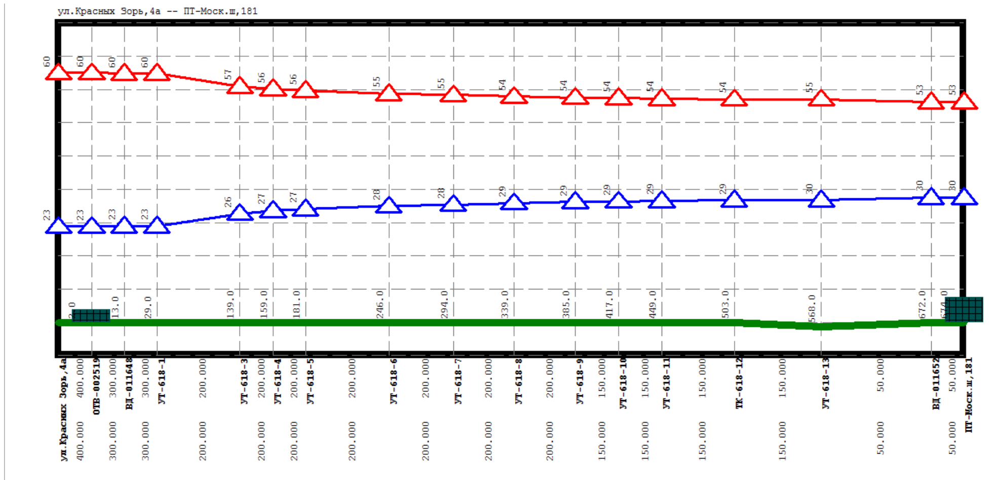
Рисунок Ошибка! Текст указанного стиля в документе отсутствует..80 Результат гидравлического расчета - график гидравлических режимов по пути теплоносителя от котельной Красных Зорь, 4а до ПТ-Моск.ш,181
