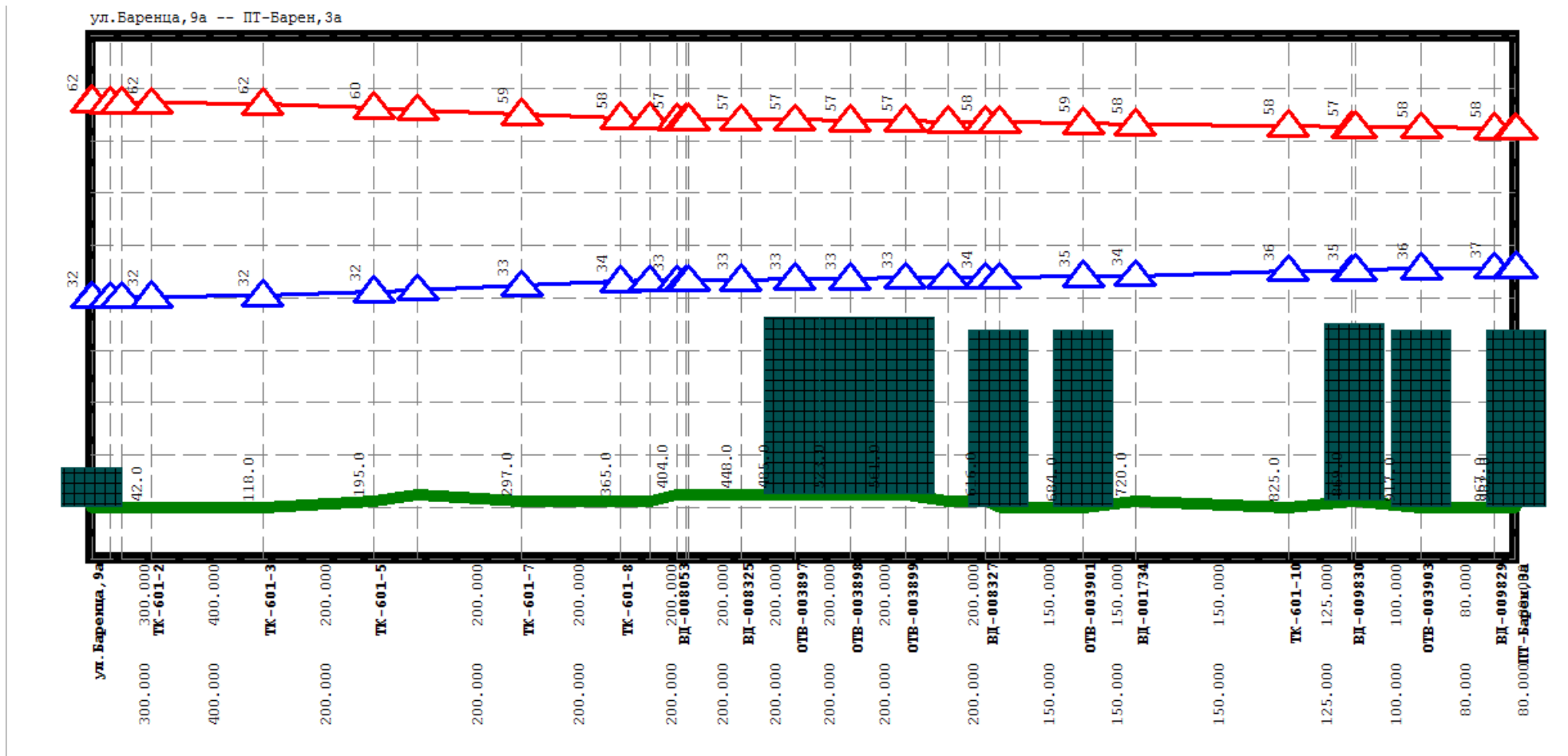
Рисунок Ошибка! Текст указанного стиля в документе отсутствует..70 Результат гидравлического расчета - график гидравлических режимов по пути теплоносителя от котельной Баренца, 9а до ПТ-Баренца
