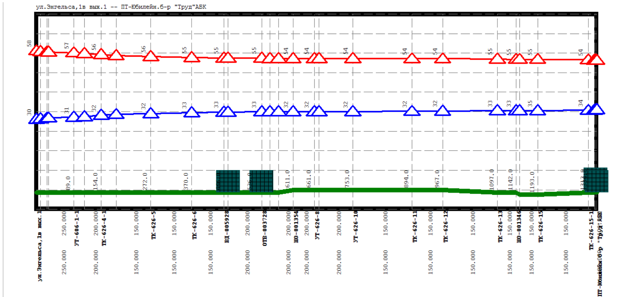
Рисунок 4.4. Результат гидравлического расчета - график гидравлических режимов по пути теплоносителя от котельной Энгельса, 1-в до ПТ-Юбилейн.б-р "Труд"АБК
