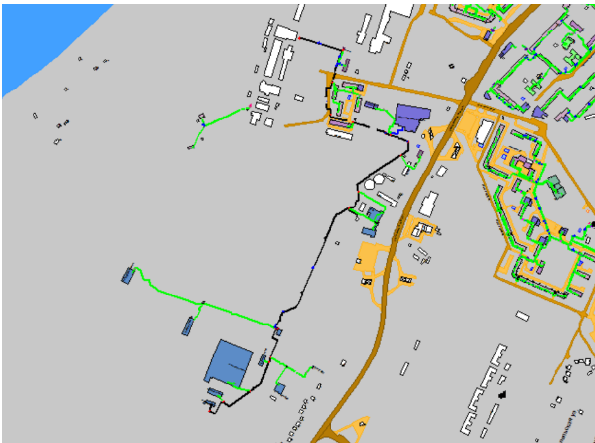
Рисунок Ошибка! Текст указанного стиля в документе отсутствует..215 Результат гидравлического расчета - расчетный путь теплоносителя от котельной Тропинина, 47 до ПТ-Гагар,121 хлор.хоз
