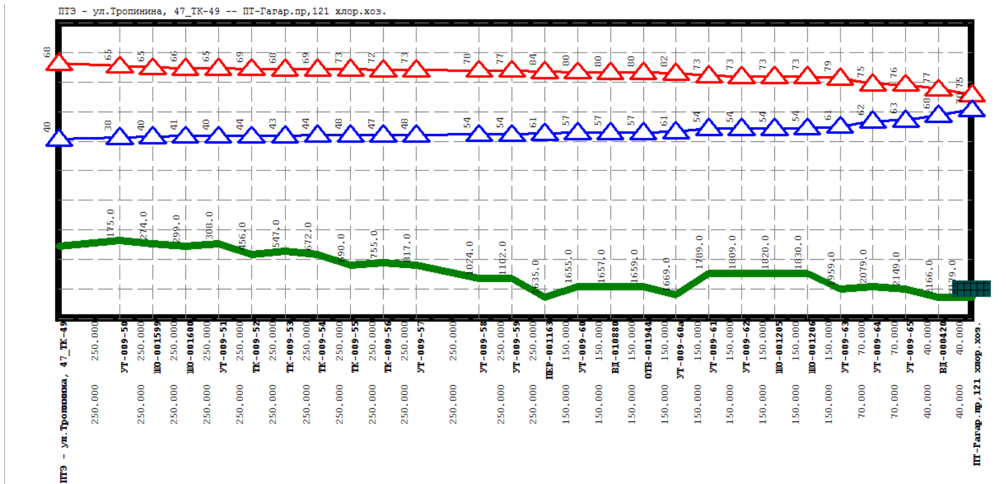
Рисунок Ошибка! Текст указанного стиля в документе отсутствует..216 Результат гидравлического расчета - график гидравлических режимов по пути теплоносителя от котельной Тропинина, 47 до ПТ-Гагар,121 хлор.хоз
