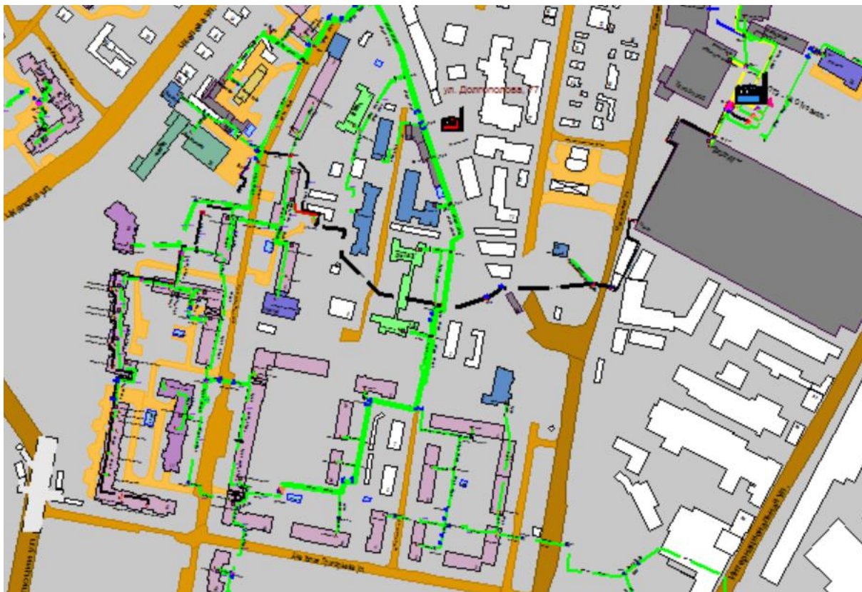
Рисунок Ошибка! Текст указанного стиля в документе отсутствует..67 Результат гидравлического расчета - расчетный путь теплоносителя от котельной Литвинова, 74 до ПТ-Октяб.рев,42 вв6
