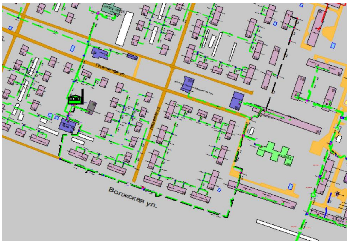
Рисунок Ошибка! Текст указанного стиля в документе отсутствует..75 Результат гидравлического расчета - расчетный путь теплоносителя от котельной Планетная, 8а до ПТ-Ясная,30а э2
