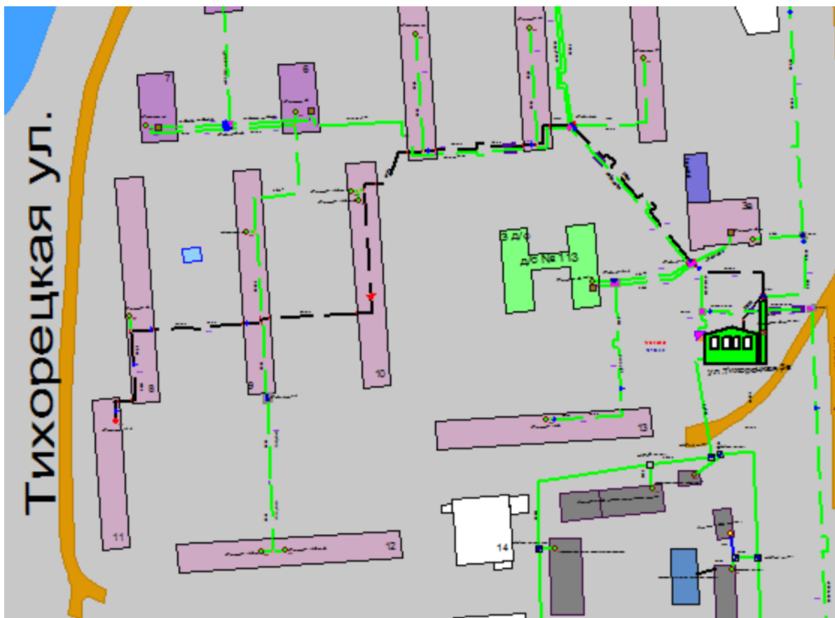
Рисунок Ошибка! Текст указанного стиля в документе отсутствует..83 Результат гидравлического расчета - расчетный путь теплоносителя от котельной Тихорецкая, 3в до ПТ-Тихор,11
