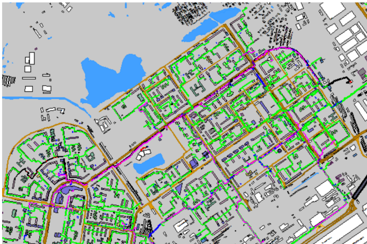
Рисунок Ошибка! Текст указанного стиля в документе отсутствует..237 Результат гидравлического расчета - расчетный путь теплоносителя от котельной Новикова-Прибоя, 18 до ПТ-Строкина,16
