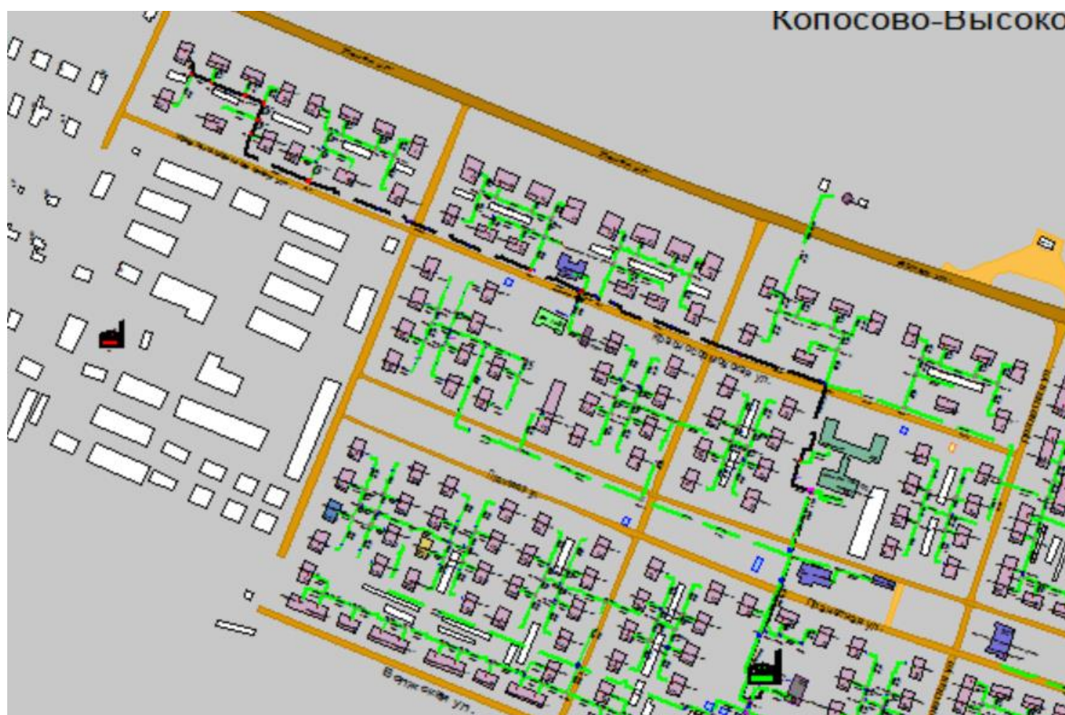
Рисунок Ошибка! Текст указанного стиля в документе отсутствует..73 Результат гидравлического расчета - расчетный путь теплоносителя от котельной Планетная, 8а до ПТ-Ясная,24
