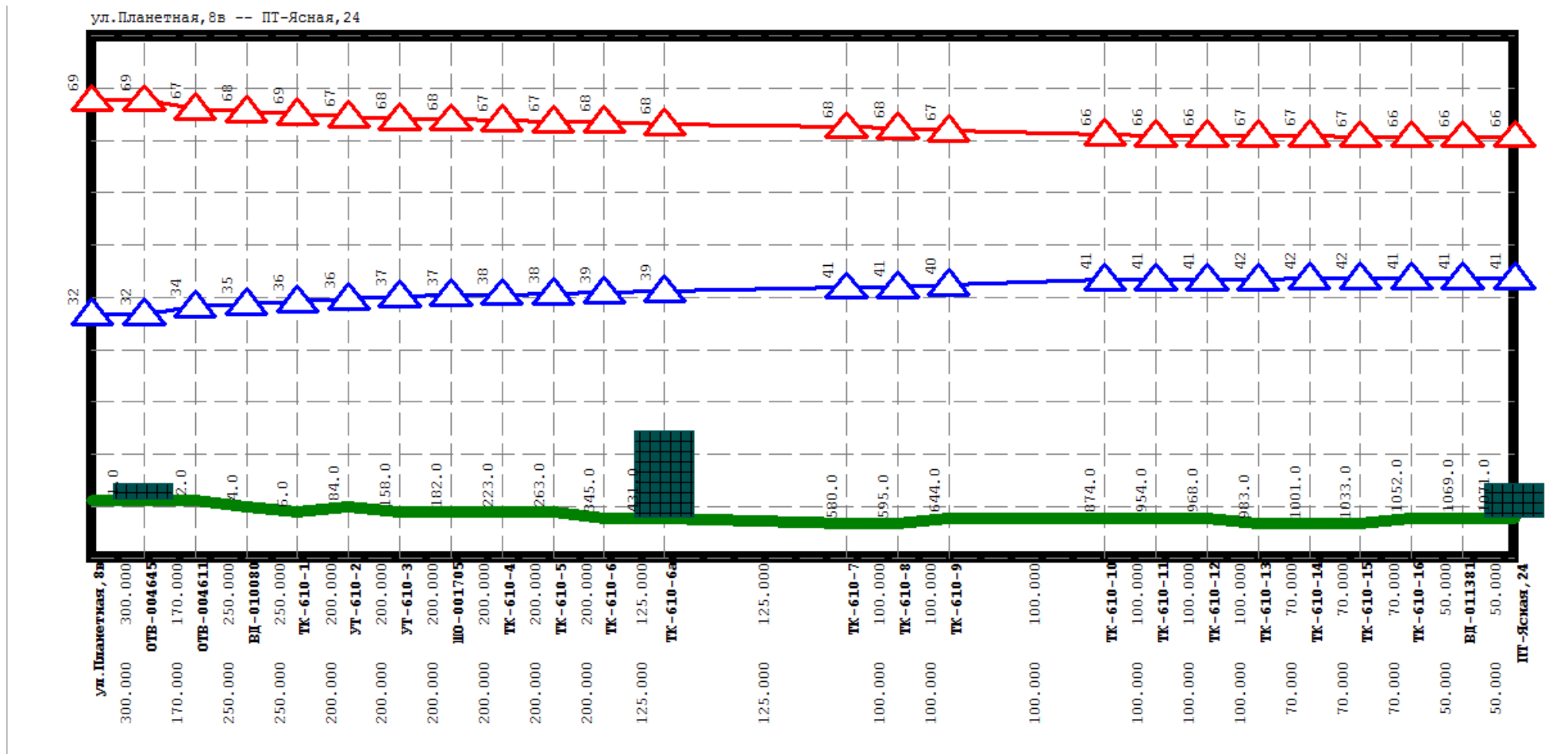
Рисунок Ошибка! Текст указанного стиля в документе отсутствует..74 Результат гидравлического расчета - график гидравлических режимов по пути теплоносителя от котельной Планетная, 8а до ПТ-Ясная,24
