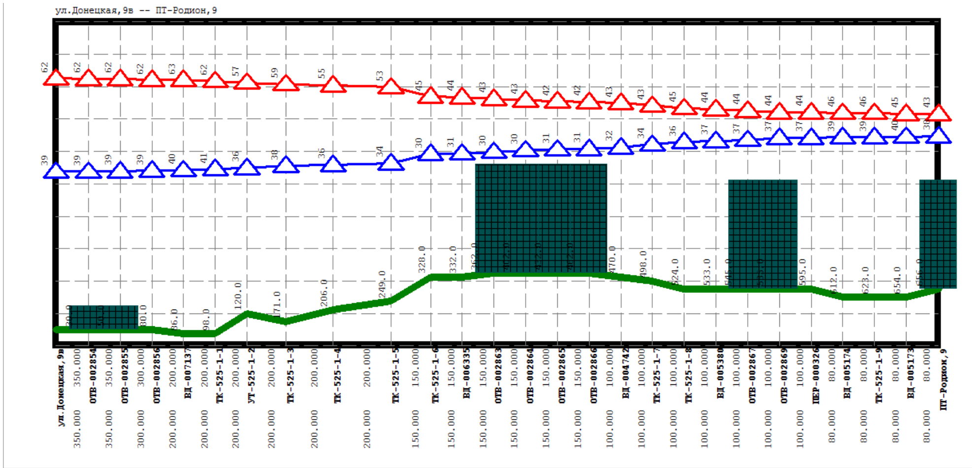
Рисунок 230 Результат гидравлического расчета - график гидравлических режимов по пути теплоносителя от котельной Донецкая, 9в до ПТ-Родион,9
