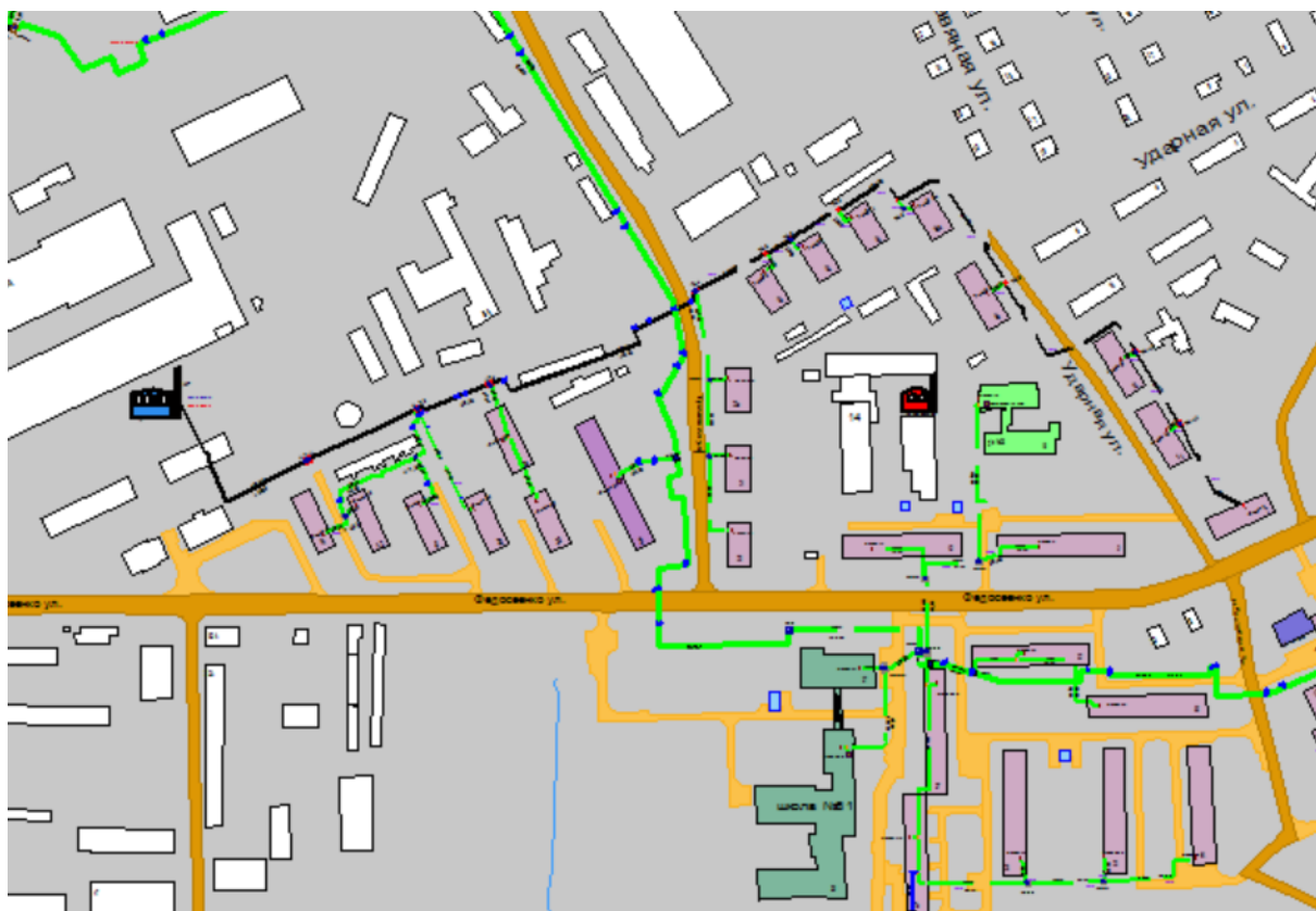
Рисунок Ошибка! Текст указанного стиля в документе отсутствует..209 Результат гидравлического расчета - расчетный путь теплоносителя от котельной Федосеенко, 44а до ПТ-Федос,7
