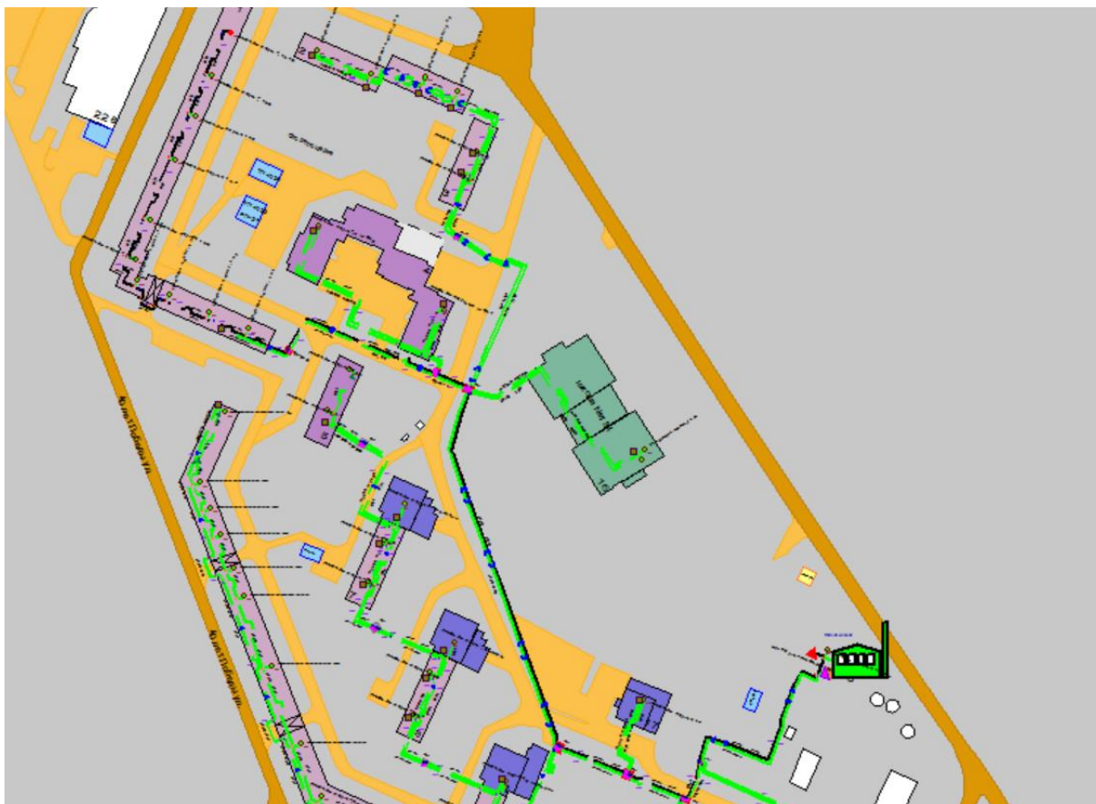
Рисунок Ошибка! Текст указанного стиля в документе отсутствует..43 Результат гидравлического расчета - расчетный путь теплоносителя от котельной 40 лет Победы, 15 до ПТ-Победы 40лет,1 э10
