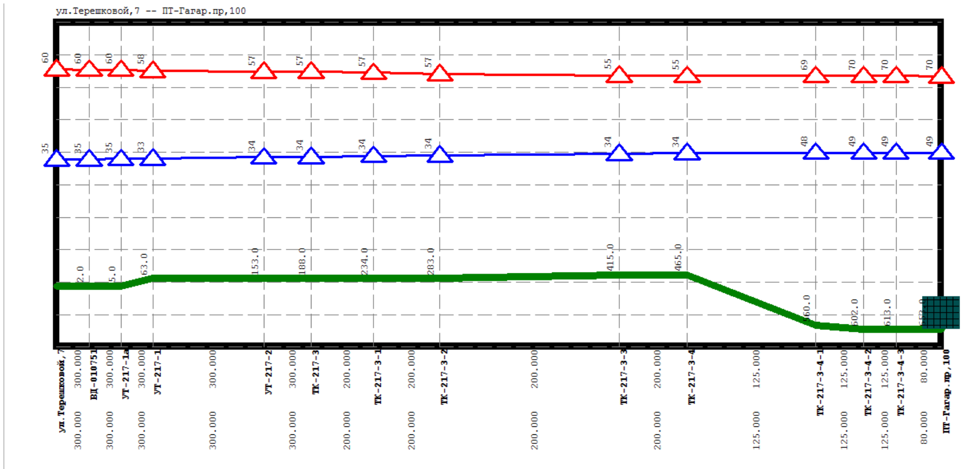
Рисунок Ошибка! Текст указанного стиля в документе отсутствует..220 Результат гидравлического расчета - график гидравлических режимов по пути теплоносителя от котельной Терешковой, 7 до ПТ-Гагар.пр,100
