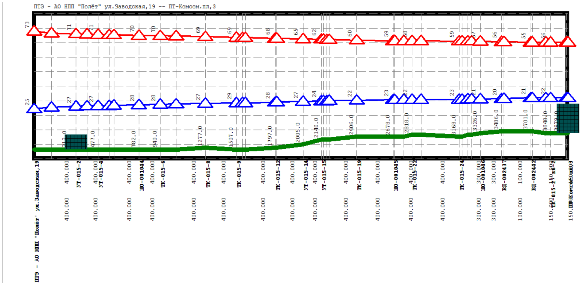
Рисунок Ошибка! Текст указанного стиля в документе отсутствует..66 Результат гидравлического расчета - график гидравлических режимов по пути теплоносителя от котельной Заводская, 19 до ПТ-Комсом.пл,3
