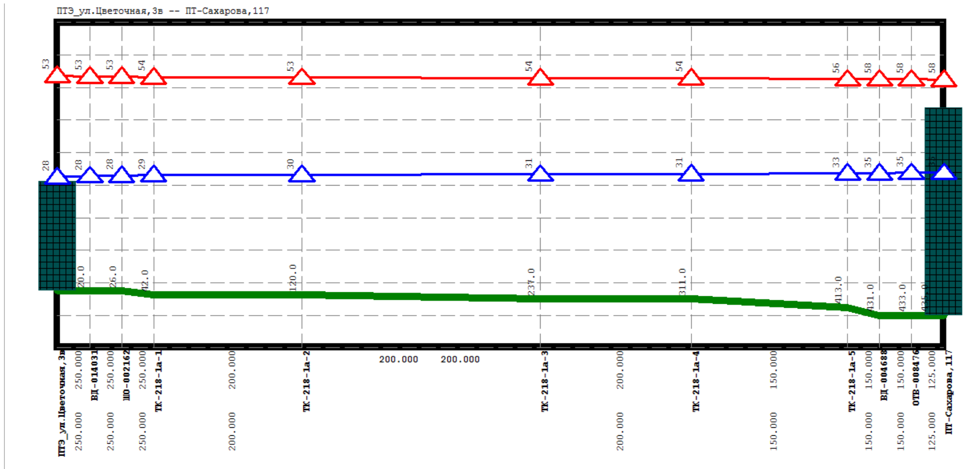
Рисунок Ошибка! Текст указанного стиля в документе отсутствует..50 Результат гидравлического расчета - график гидравлических режимов по пути теплоносителя от котельной Цветочная, 3-а до ПТ-Сахарова, 117
