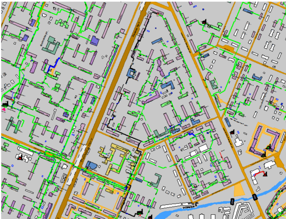
Рисунок Ошибка! Текст указанного стиля в документе отсутствует..13 Результат гидравлического расчета - расчетный путь теплоносителя от котельной Геройская, 11-а до ПТ-пр. Ленина, 38
