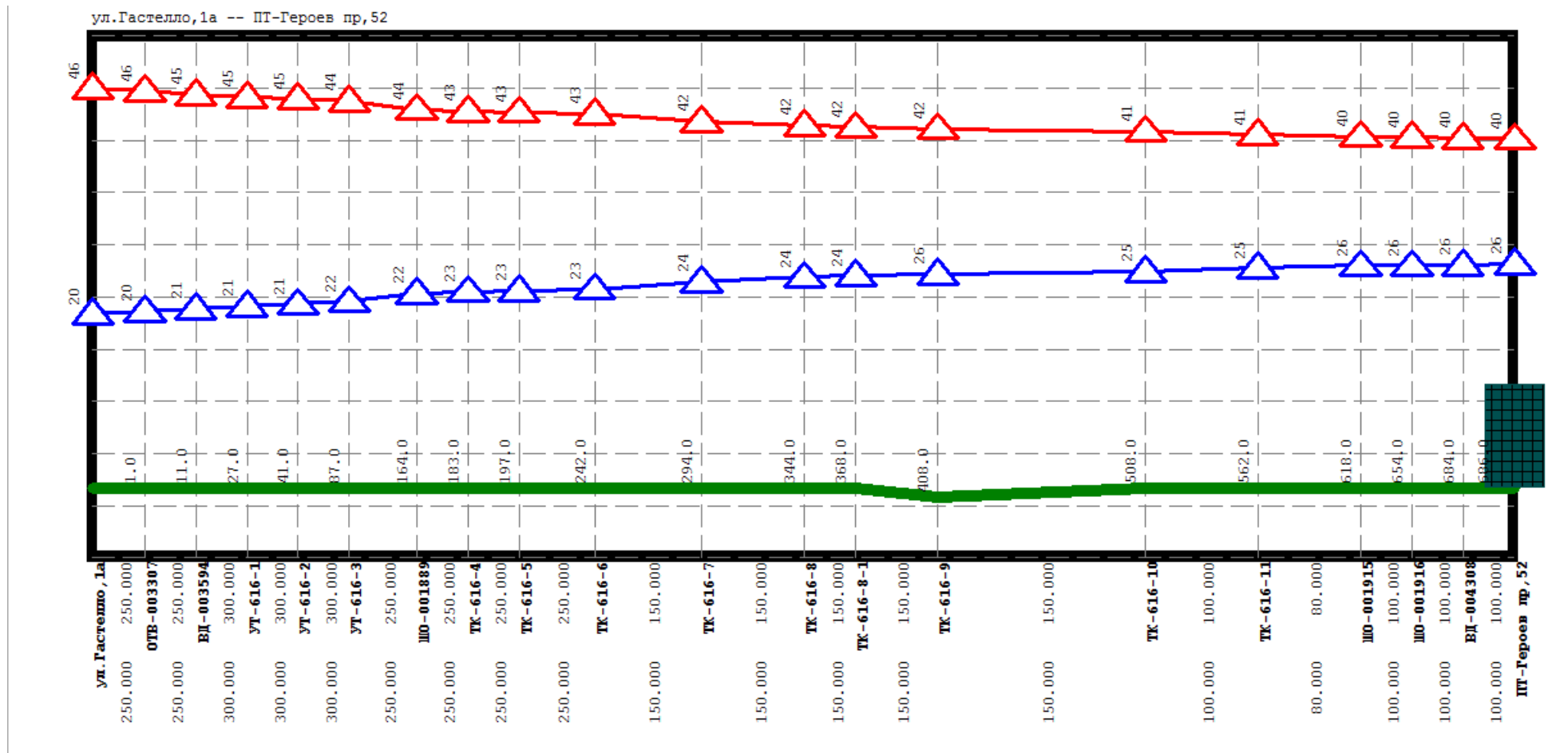
Рисунок Ошибка! Текст указанного стиля в документе отсутствует..22 Результат гидравлического расчета - график гидравлических режимов по пути теплоносителя от котельной Гастелло, 1-а до ПТ-Героев пр,52
