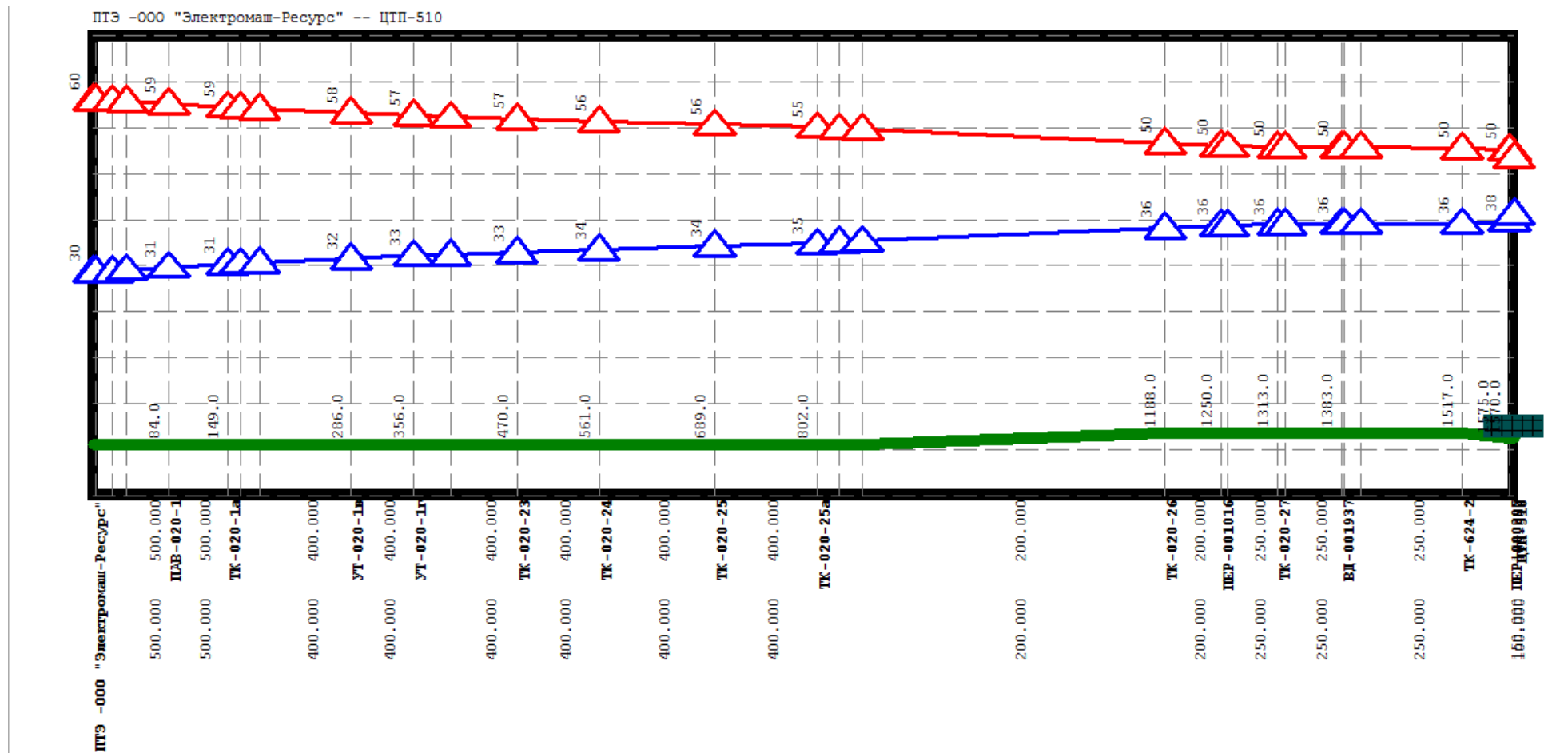
Рисунок Ошибка! Текст указанного стиля в документе отсутствует..212 Результат гидравлического расчета - график гидравлических режимов по пути теплоносителя от котельной Федосеенко, 64 до ЦТП-510
