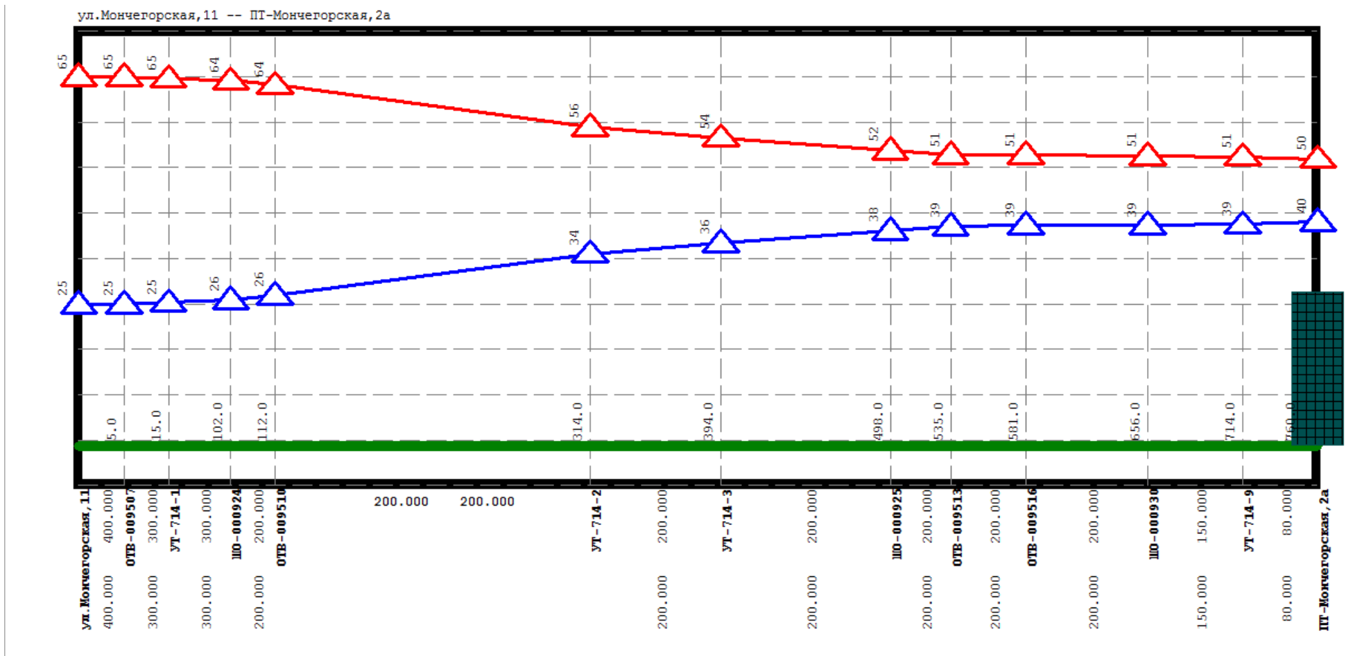
Рисунок Ошибка! Текст указанного стиля в документе отсутствует..208 Результат гидравлического расчета - график гидравлических режимов по пути теплоносителя от котельной Мончегорская, 11 до ПТ-Мончегорская,2а
