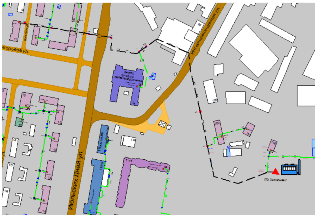
Рисунок Ошибка! Текст указанного стиля в документе отсутствует..235 Результат гидравлического расчета - расчетный путь теплоносителя от котельной Интернациональная, 95 до ПТ-Вольск,11
