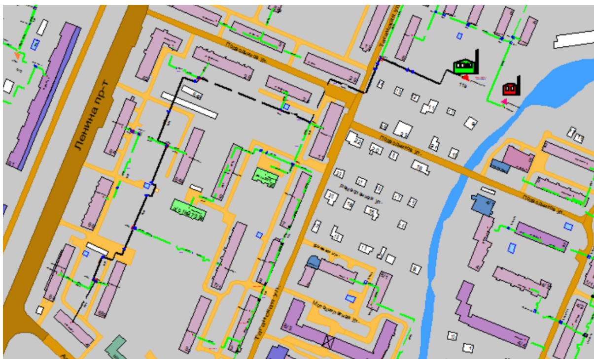
Рисунок Ошибка! Текст указанного стиля в документе отсутствует..11 Результат гидравлического расчета - расчетный путь теплоносителя от котельной Геройская, 11-а до ПТ-Адм.Нахим, 4
