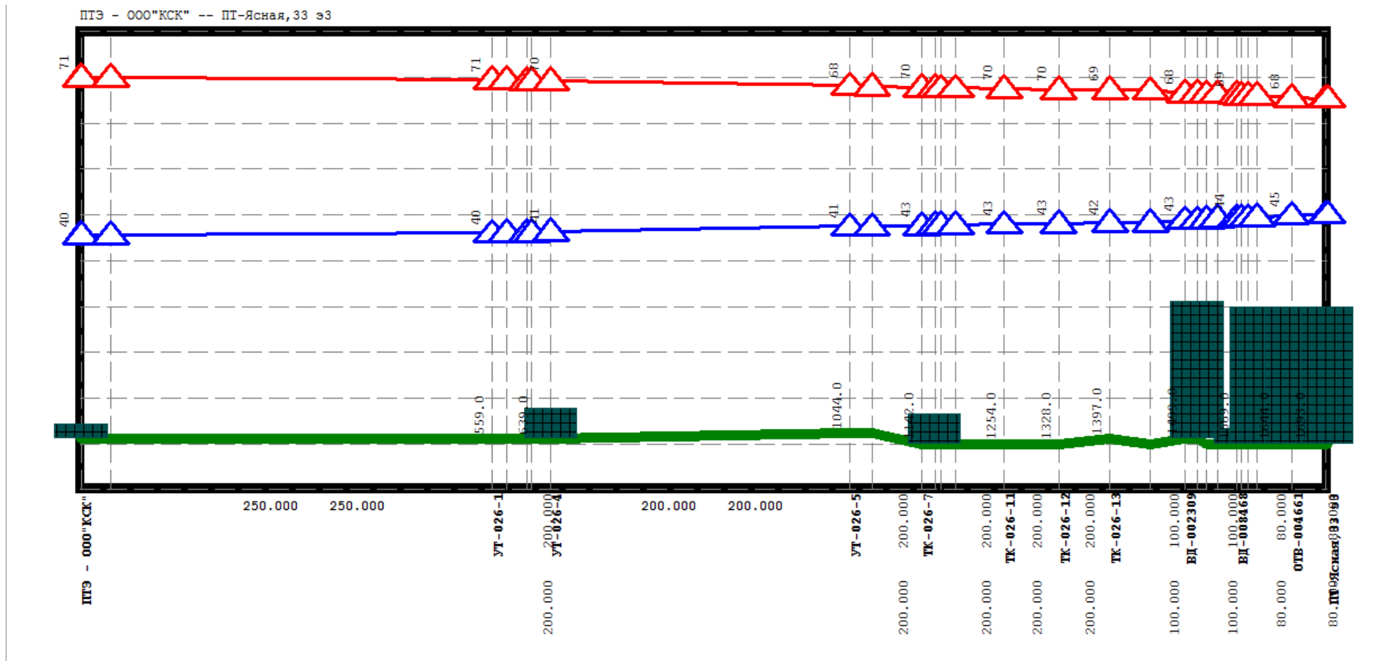
Рисунок Ошибка! Текст указанного стиля в документе отсутствует..60 Результат гидравлического расчета - график гидравлических режимов по пути теплоносителя от котельной Зайцева, 31 до ПТ-Ясная, 33 эЗ
